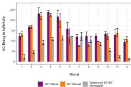
2_ Gemessene Stromerträge der alpinen Solaranlage Davos-Totalp im Vergleich zu einer Anlage auf einem Dach in Wädenswil – im Betrachtungsraum vom 1. Oktober 2020 bis zum 31. August 2023. Die durchschnittlichen Monatserträge sind als Säulen dargestellt – mit den jeweiligen Maximal- und Minimalwerten als Doppel-T.
